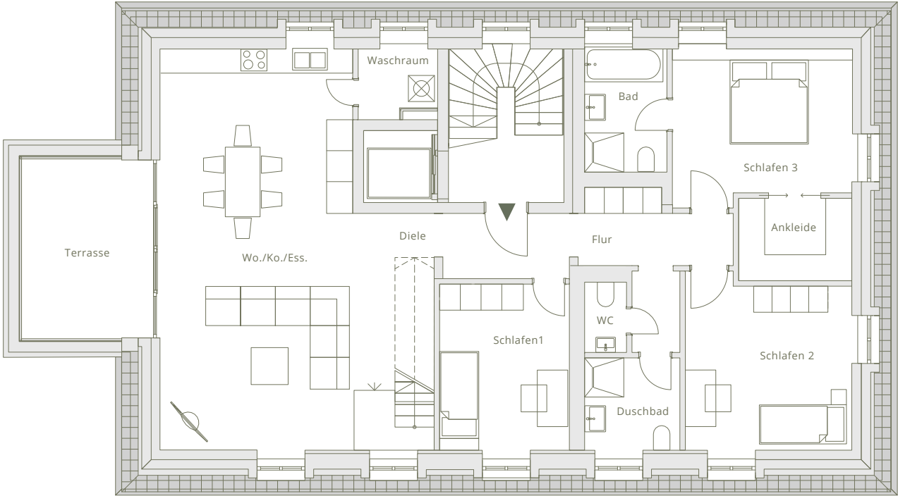
DACHGESCHOSS
